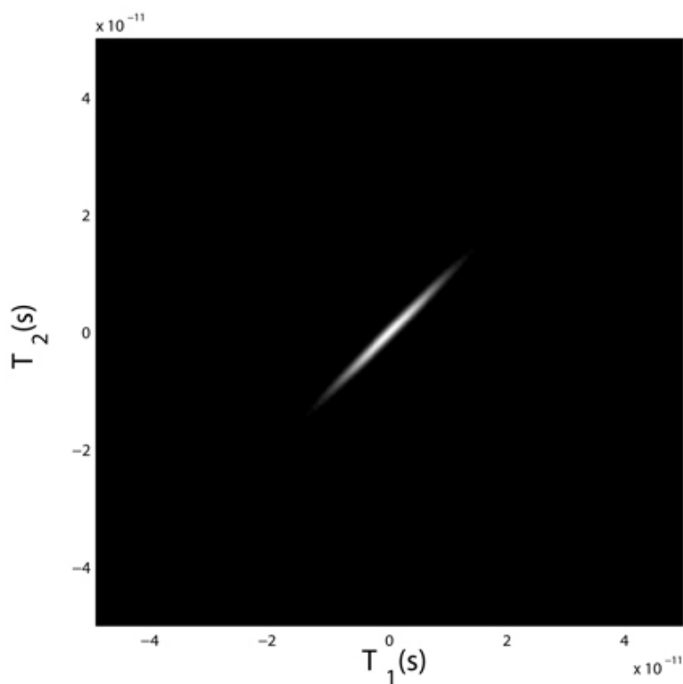
Figure 4 : Fonction de corrélation d'ordre 2
