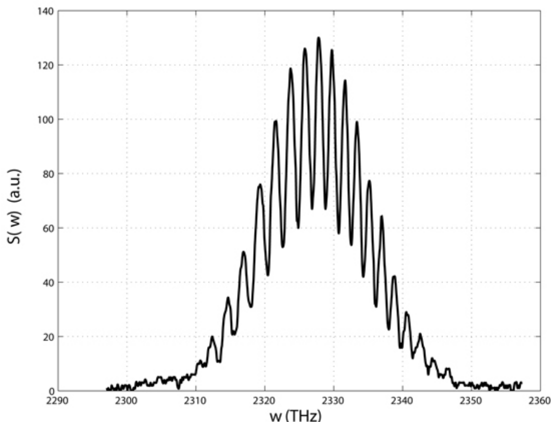
Figure 11 : Interférogramme expérimental SPIRIT
