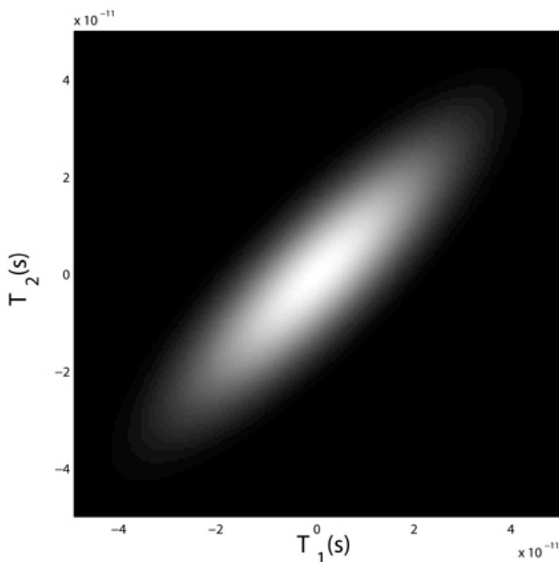
Figure 5 : Fonction de corrélation d'ordre 2 après propagation
