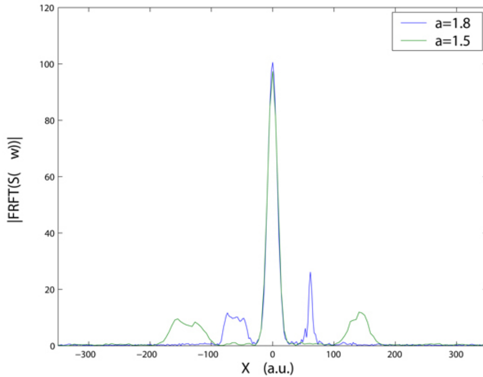
Figure 12 : 2 transformées de Fourier fractionnaires d'ordres différents de l'interférogramme SPIRIT expérimental
