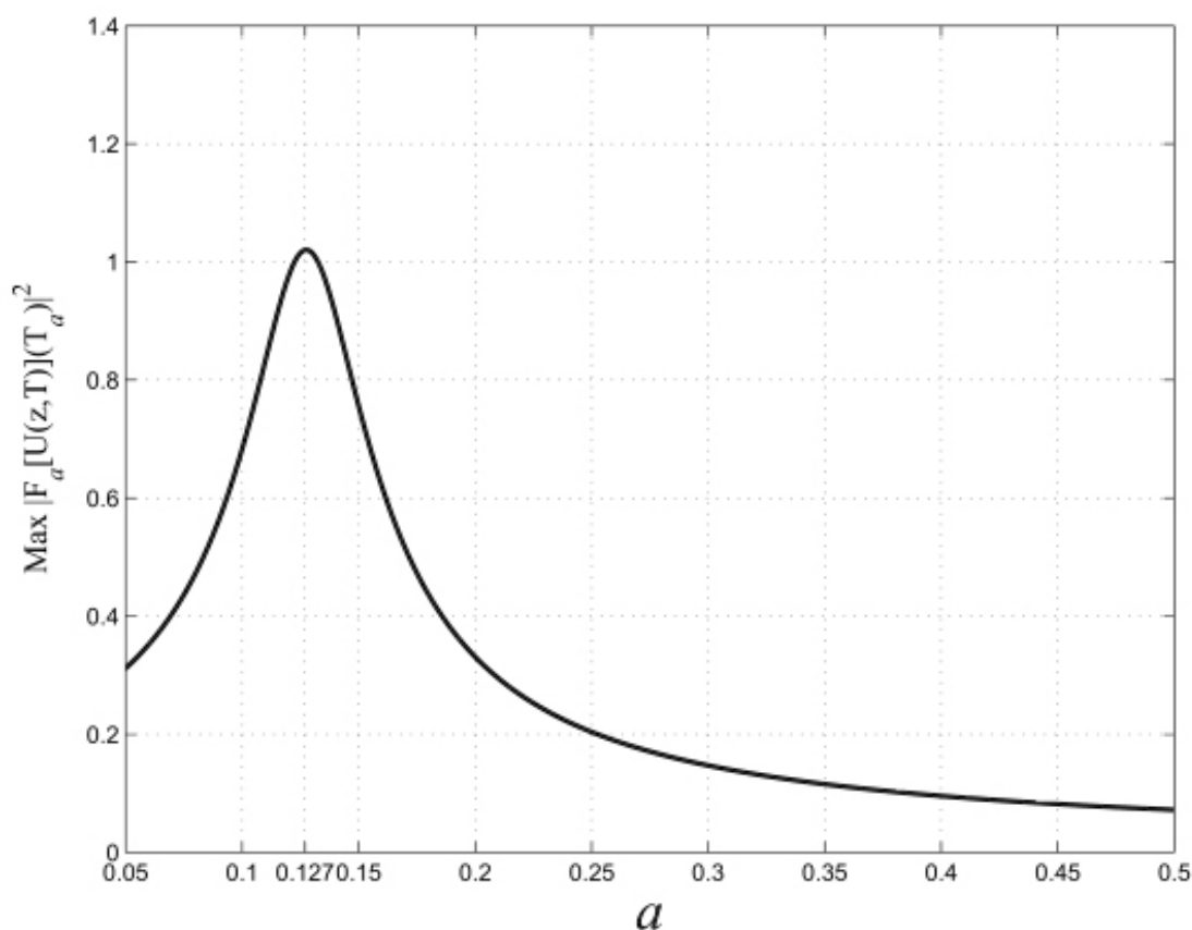
Figure 6 : Reconnaissance d'une dérive de fréquence linéaire
