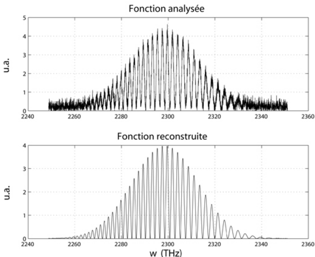
Figure 14 : Signal bruité puis reconstruit
