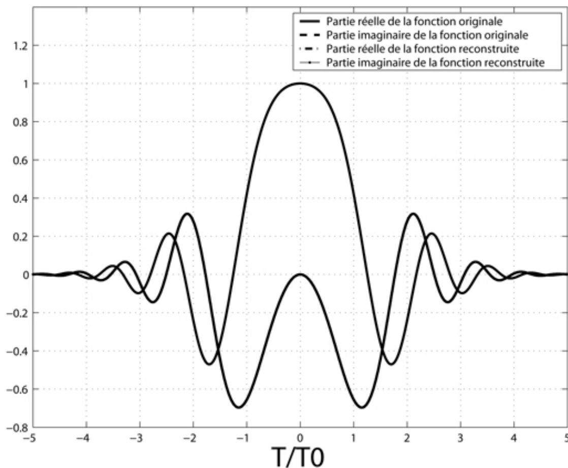
Figure 10 : Signal initial et reconstruit
