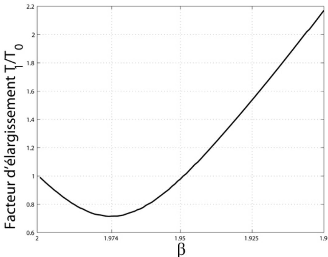
Figure 3 : Compression d'une impulsion initialement chirpée
